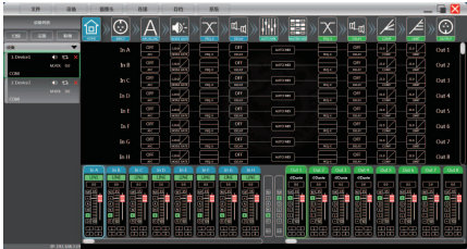
软件界面
